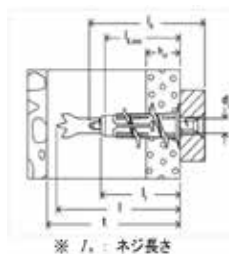
※ l 1 ：ネジ長さ
